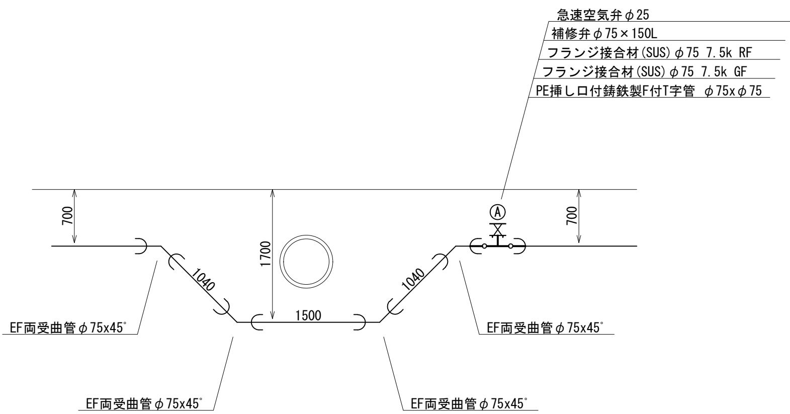
b - b 断面図
