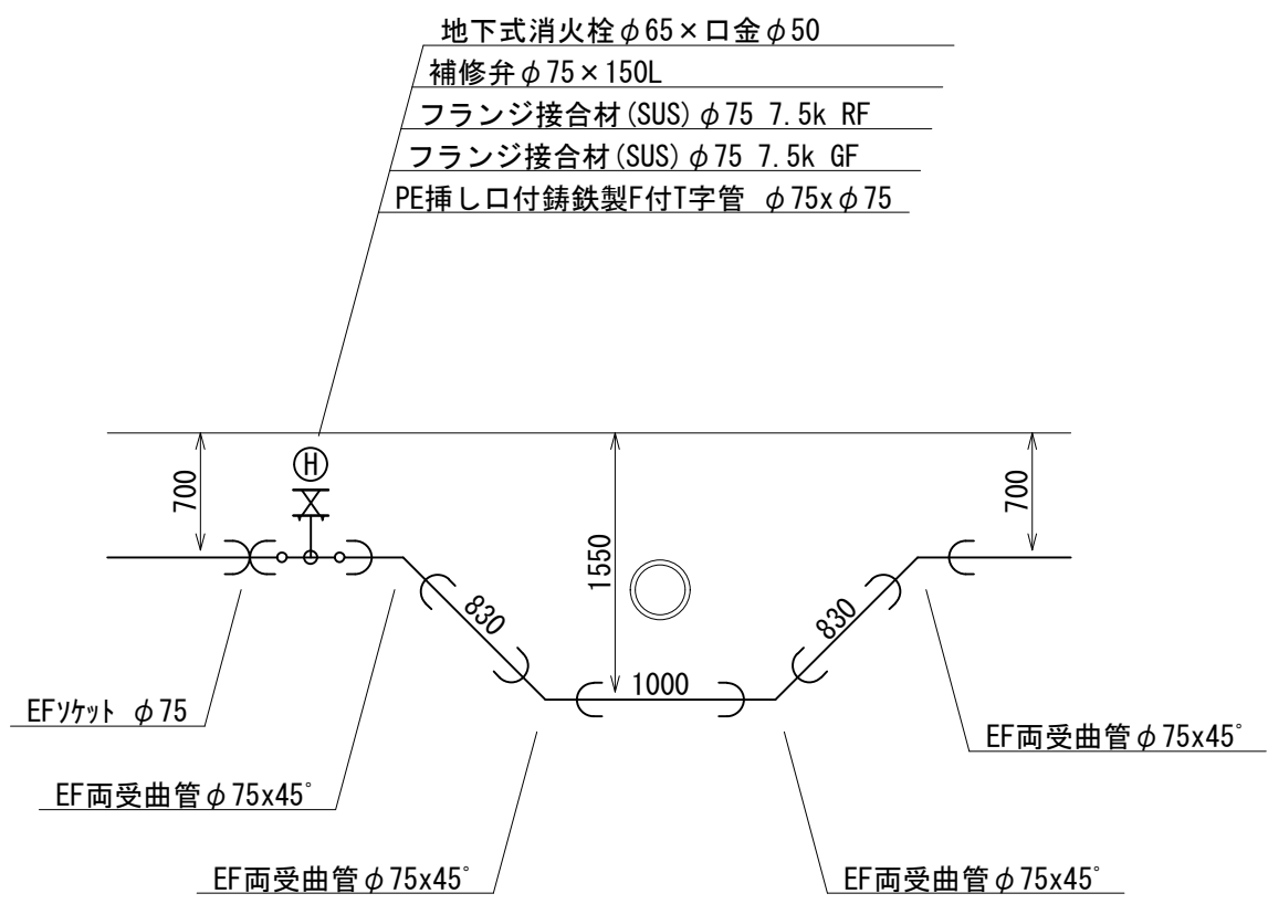
d - d 断面図
