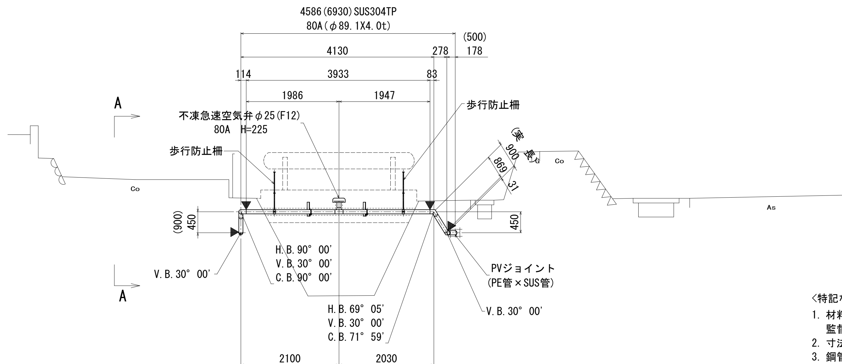
側面図
