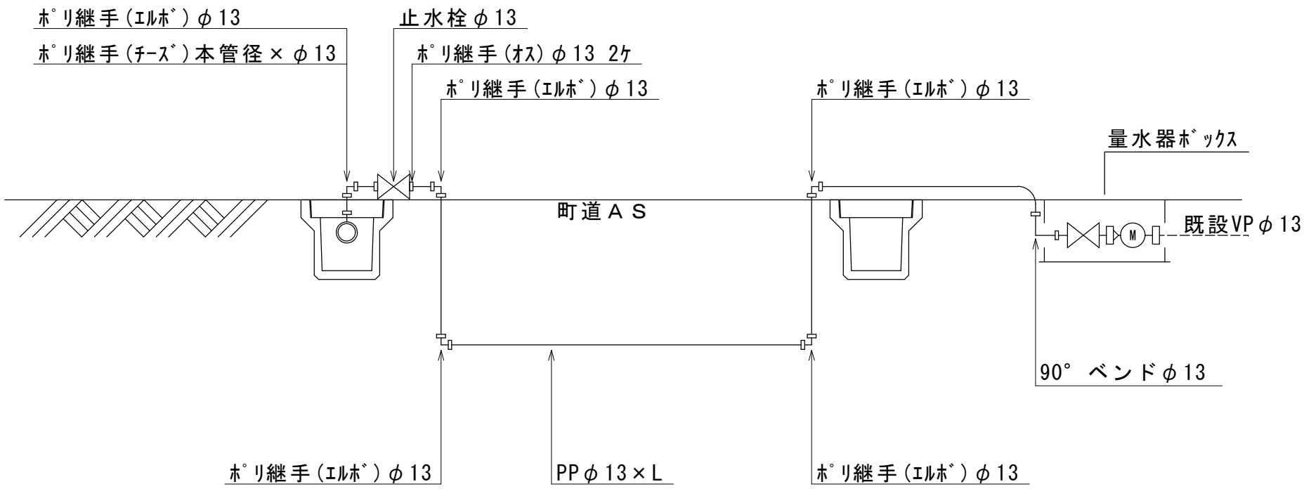
仮設給水切替標準図 (本管HPPE:複数件取出し)
