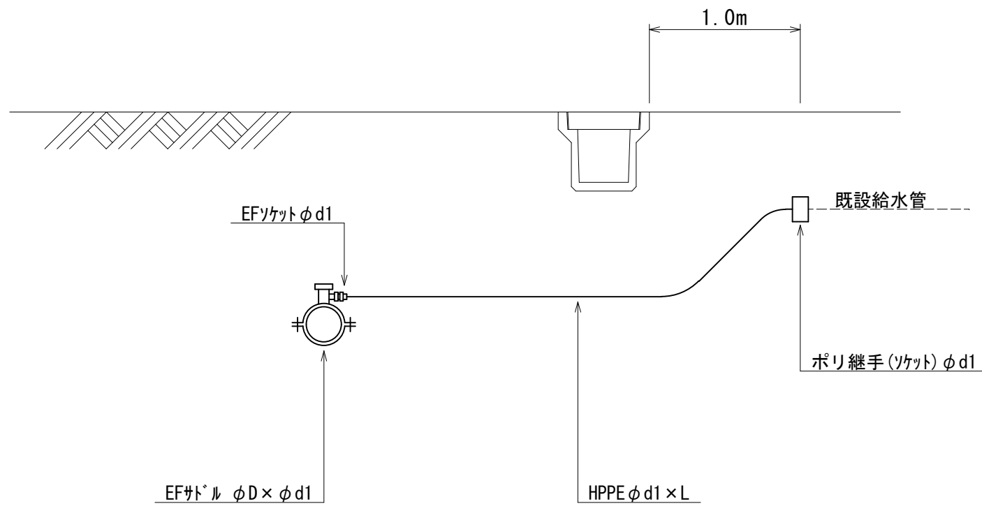
給水切替標準図 (量水器移設)
