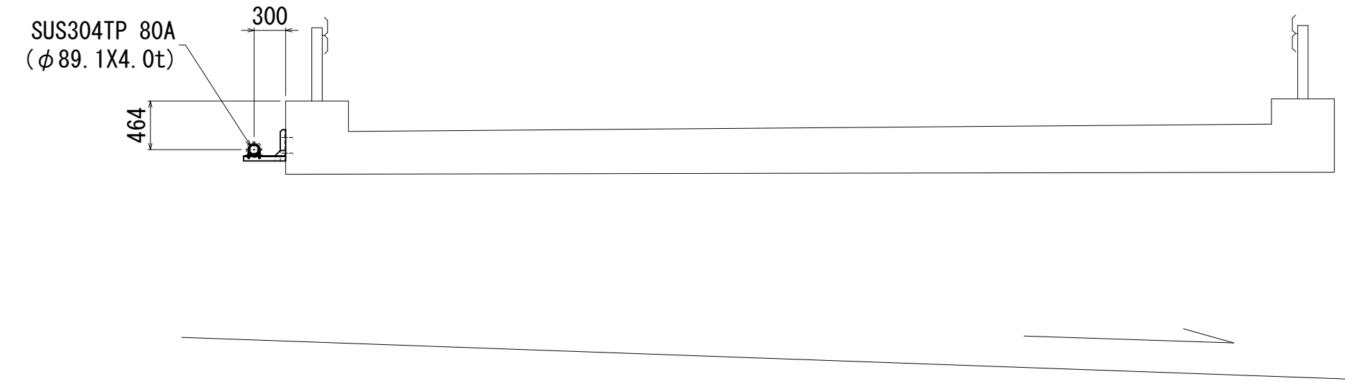
断面図
