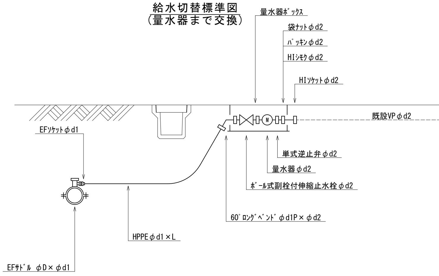
給水切替標準図 (量水器交換)
