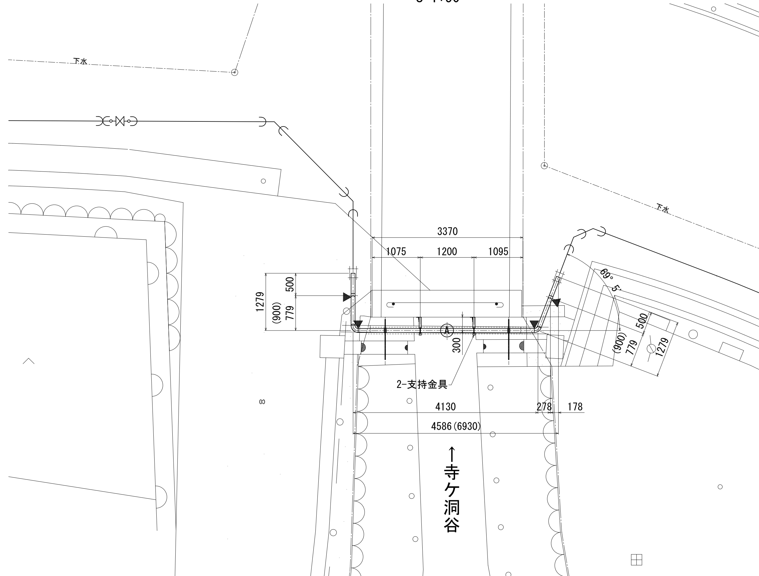
平面図
