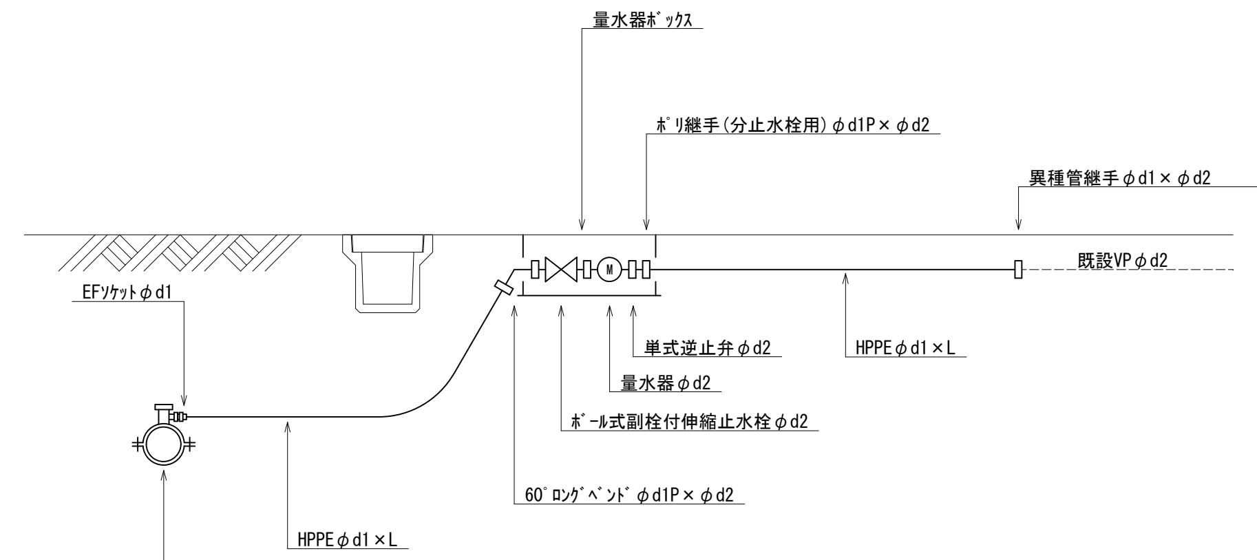
給水切替標準図 (給水管 φ30)
