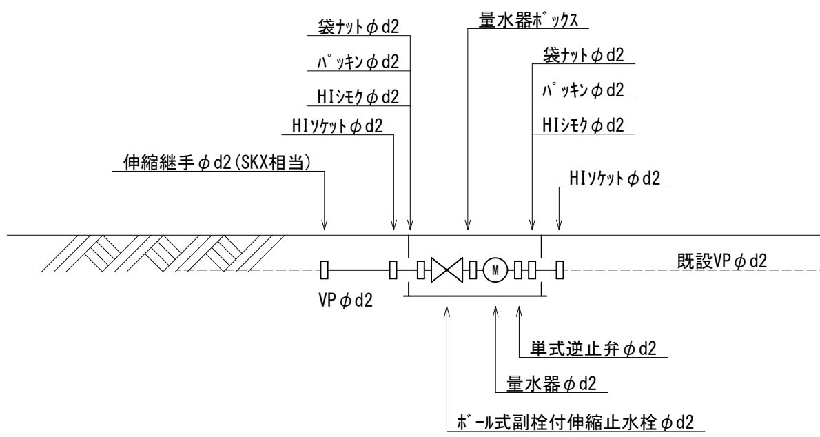
給水切替標準図 (量水器交換)
