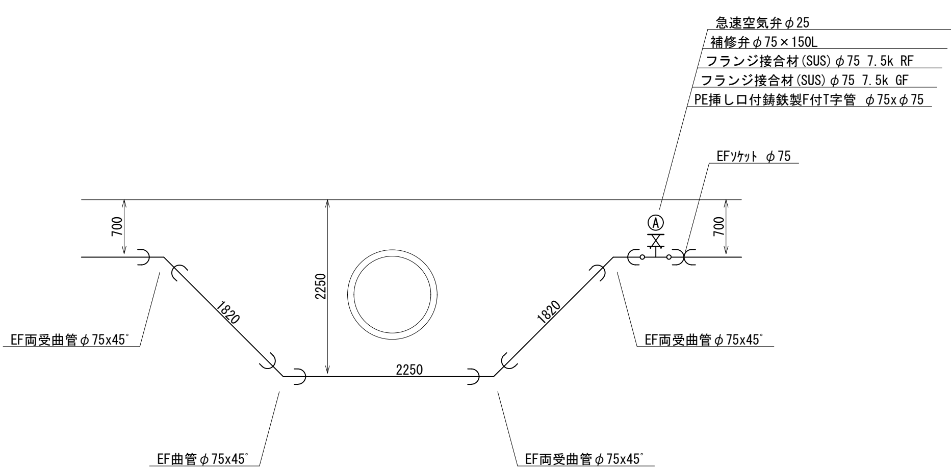
c - c 断面図
