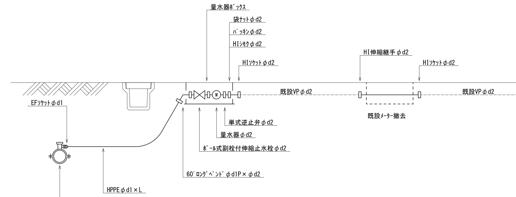
給水切替標準図 (給水管 φ30)
