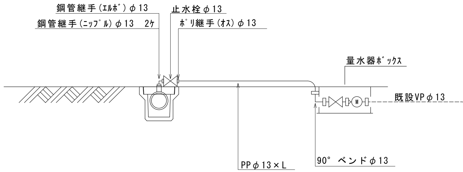
仮設給水切替標準図 (本管HPPE:1件取出し)
