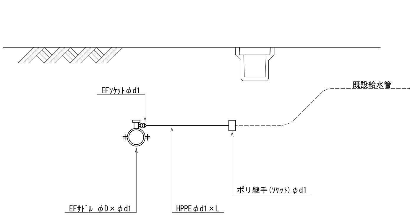
給水切替標準図 (量水器移設)
