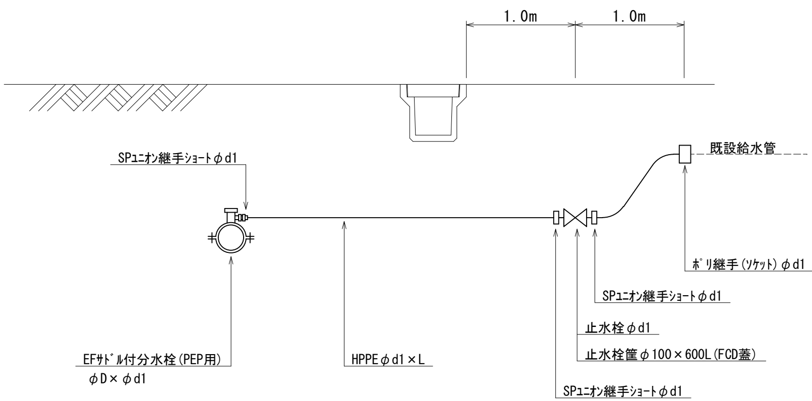
給水切替標準図 (給水管 φ30)
