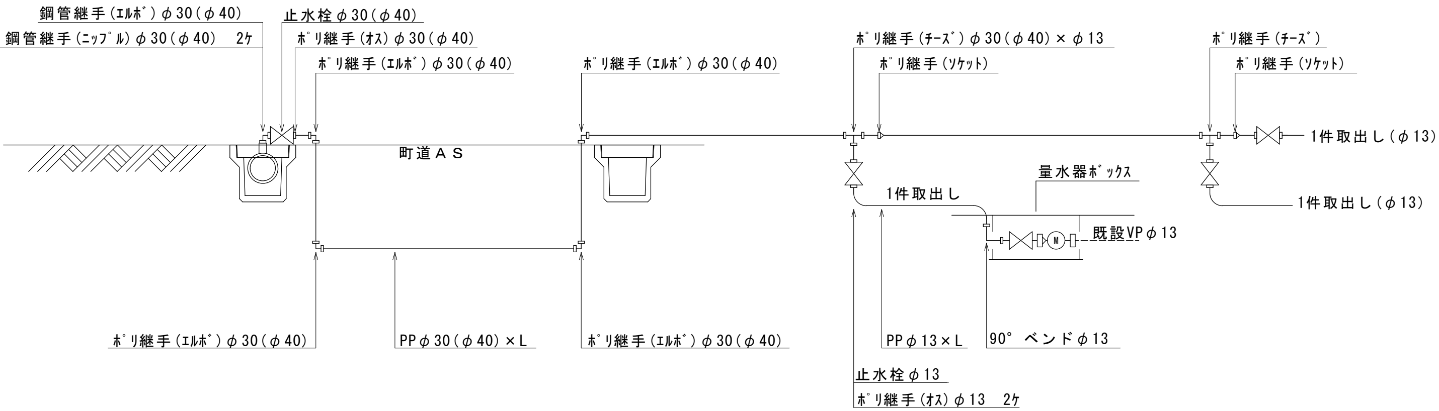
仮設給水切替標準図 (本管HPPE:複数件取出し)
