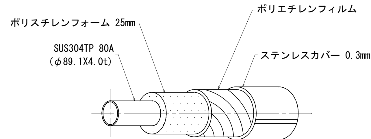
80A保温管詳細図
