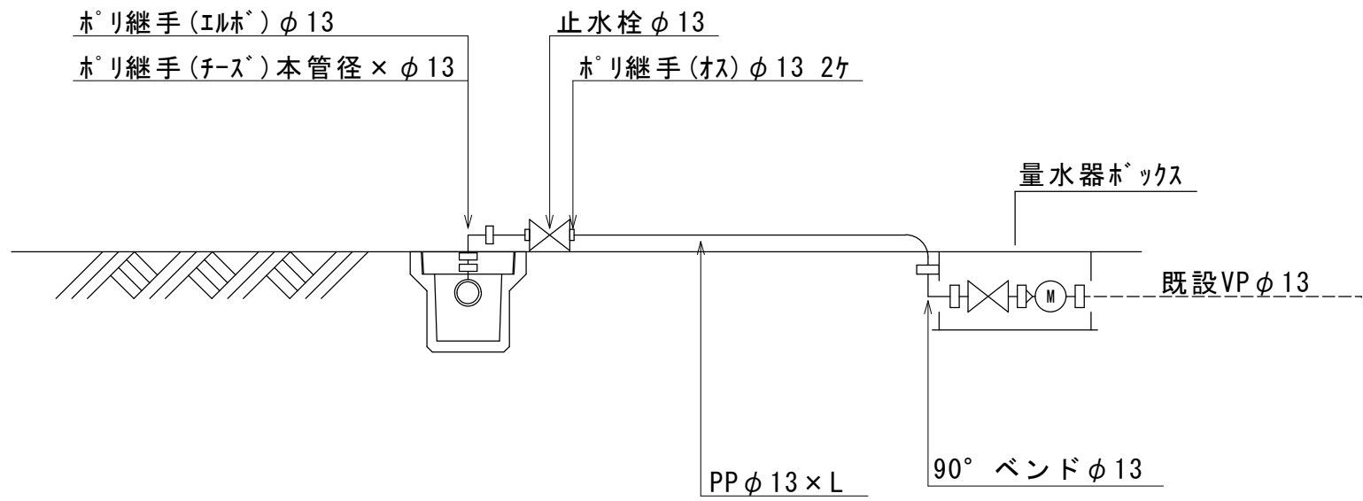
仮設給水切替標準図 (本管PEP:1件取出し)
